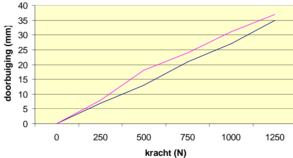
doorbuigingsvergelijk Test 1
