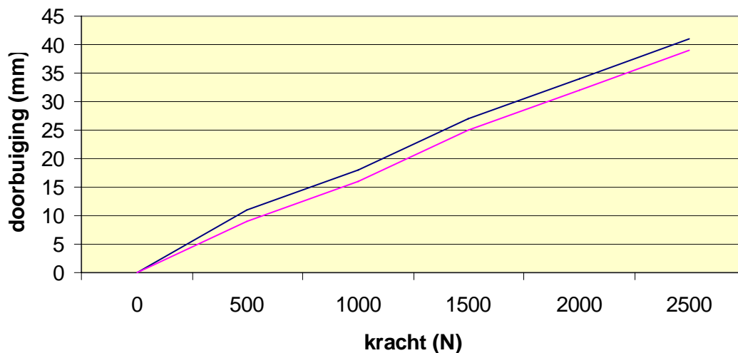
doorbuigingsvergelijk Test 2
